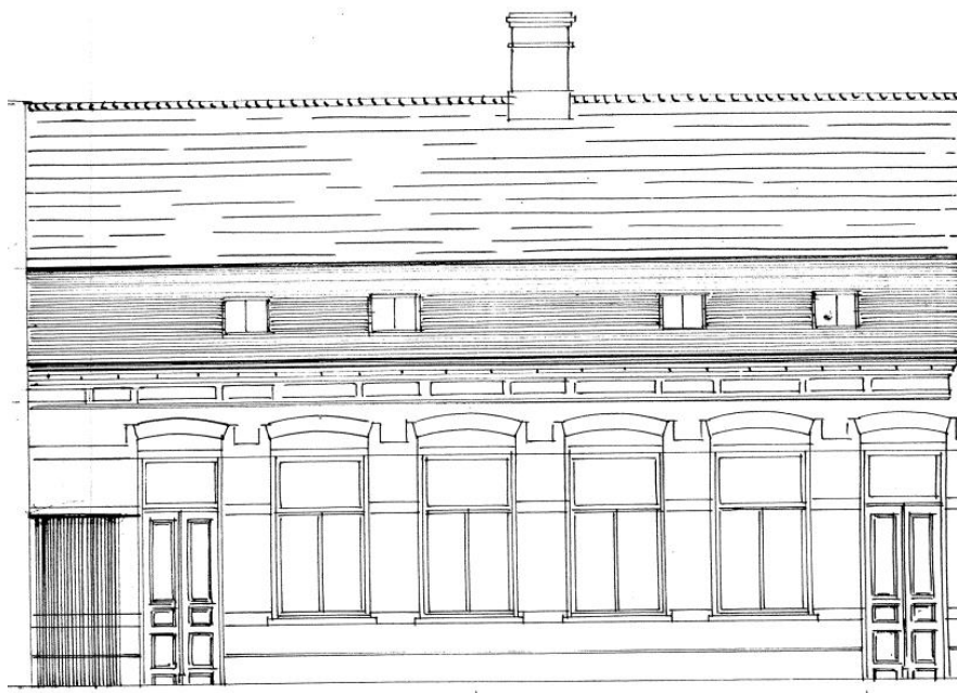
'Plan voor twee woonhuizen voor den heer Joz. vd Biggelaar te Hilvarenbeek' (1927), Varkensmarkt 14 en 16
